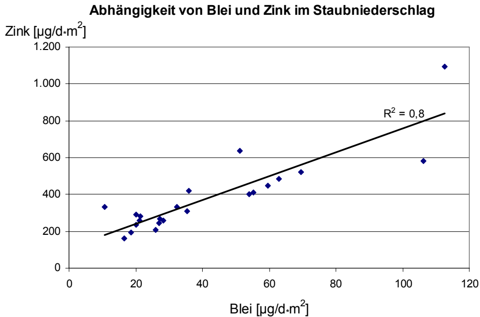
Abb. 8: Abhängigkeit der für Stahlwerke typischen Stoffe Blei und Zink im Staubbiederschlag in Riesa
