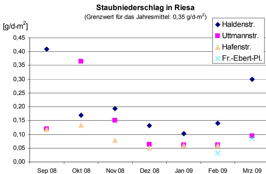
Abb. 5: Staubniederschlag in Riesa von September 2008 bis März 2009
