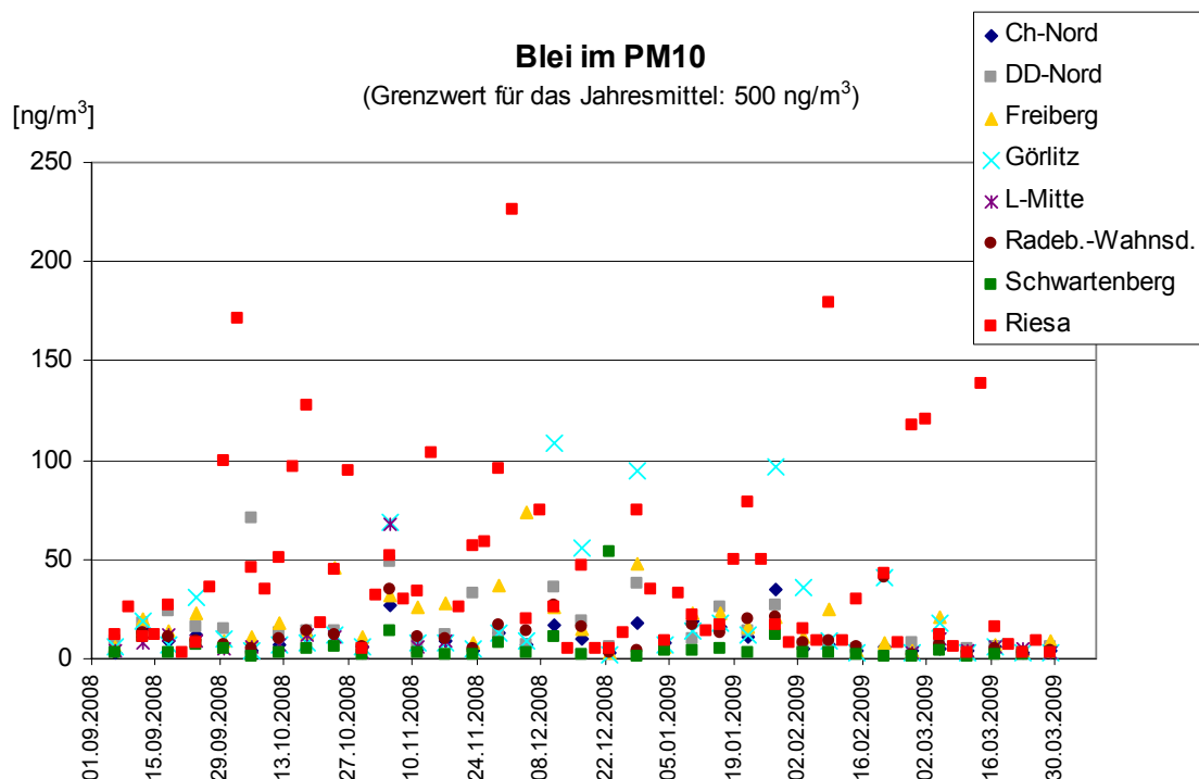
Abb. 2: Konzentration von Blei im PM10 an verschiedenen Messstationen in Sachsen September 2008 bis März 2009
