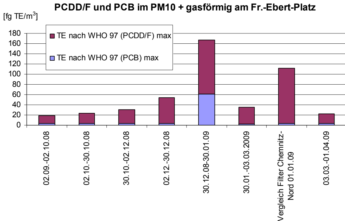
Abb. 4: PCDD/F und PCB im PM10 und gasförmig in Riesa bzw. nur im PM10 (Stichprobe vom 01.01.09 in Chemnitz-Nord)
