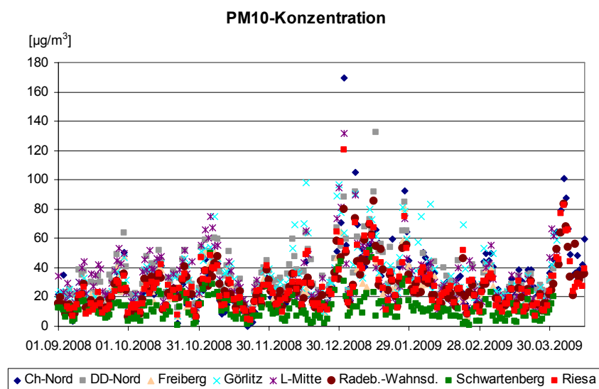
Abb. 1: PM10-Konzentration an verschiedenen Messstationen in Sachsen September 2008 bis März 2009
